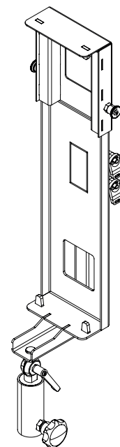
Abbildung Vario System inkl. Klemmträger und Stativaufnahme
